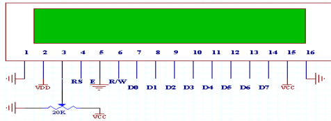
Gambar 1. Pin LCD ke Mikrokontroler [Judul Gambar: Times New Roman 8 italic centre ]
